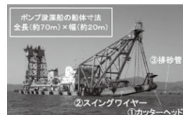
▲ポンプ浚渫船
