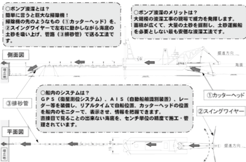
ポンプ浚渫のイメージ図▶
