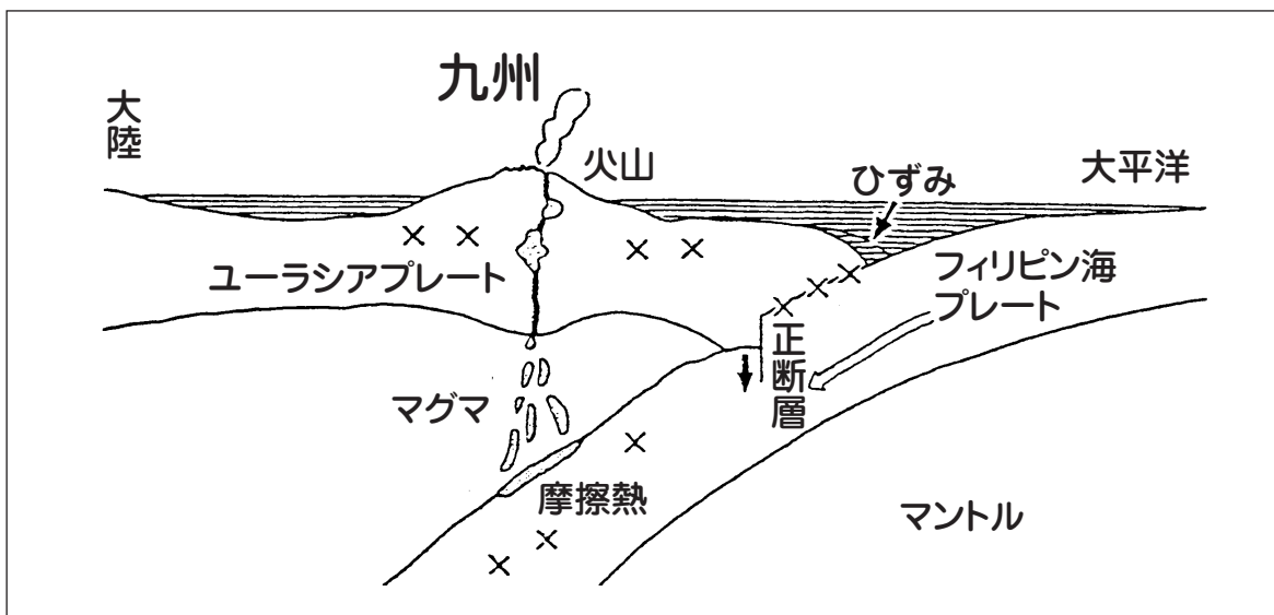
九州付近の地震と火山のイメージ図（×は震源地）
