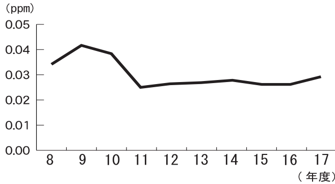
●表6 年平均値の経年変化
