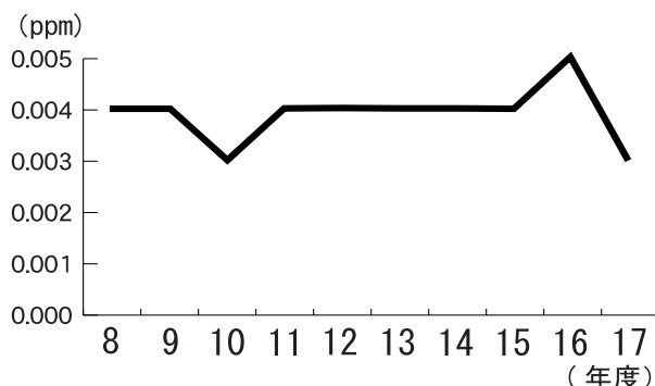
●表2 年平均値の経年変化
