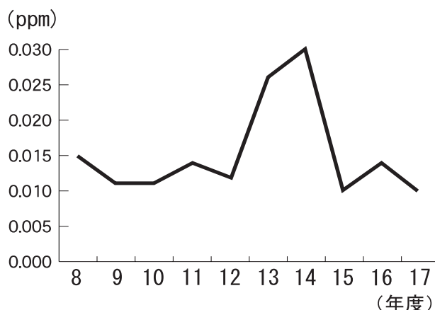
●表4 年平均値の経年変化
