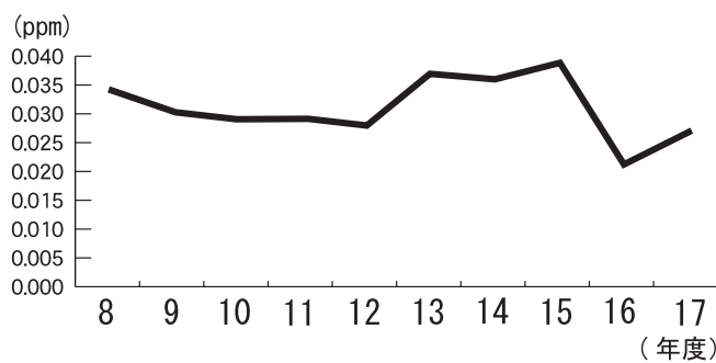
●表8 年平均値の経年変化
