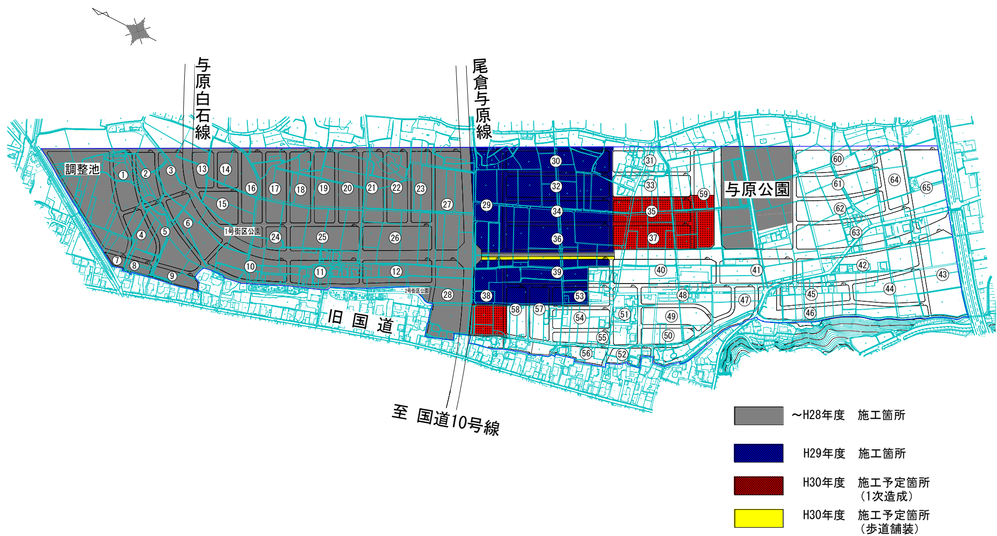
H30年度 工事予定箇所図
