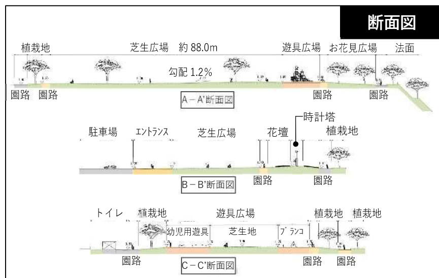
・芝生広場の勾配1.2%：100m進むと1.2m登る（角度0.688度）
